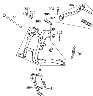
F16 Stand/Kick Starter Arm
